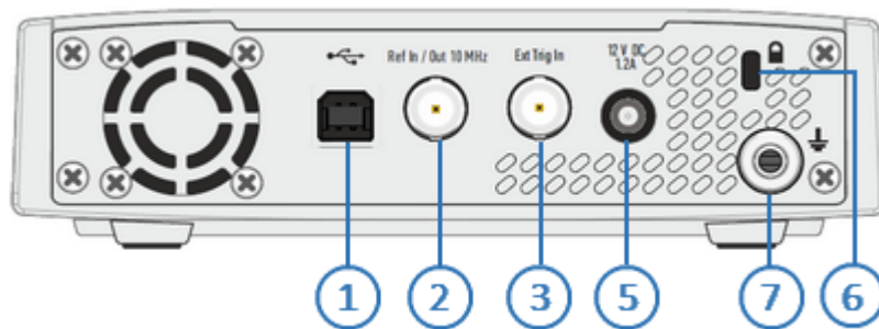
Рисунок 18 – Задняя панель
